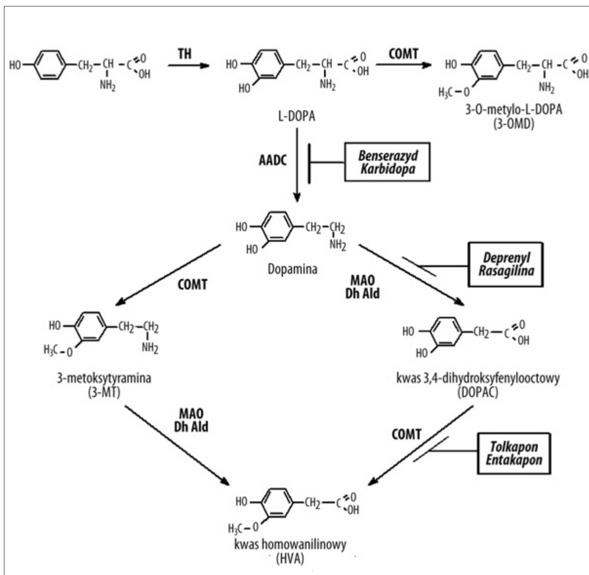
Ryc. 1. Biosynteza L-DOPA i dopaminy oraz główne drogi przemian tych związków w ośrodkowym układzie nerwowym. W prostokątnych ramkach wpisano nazwy stosowanych w leczeniu inhibitorów enzymów katalizujących dany etap szlaku; AADC – dekarboksylaza DOPA, COMT – o-metylotransferaza katecholowa, Dh Ald – mitochondrialna dehydrogenaza aldehydowa, MAO – oksydaza monoaminowa, TH – hydroksylaza tyrozynowa, benserazyd oraz karbidopa – inhibitory AADC, deprenyl oraz rasagilina – inhibitory MAO B, entapon oraz tolkapon – inhibitory COMT
