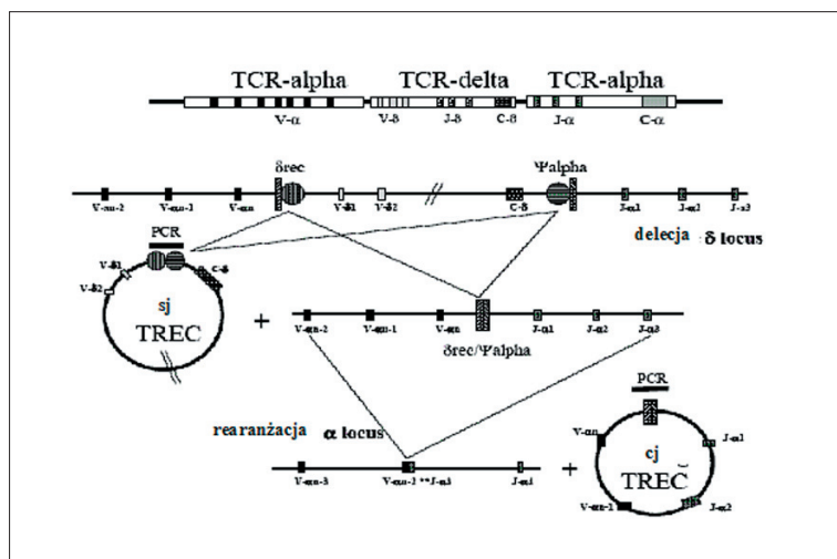
Ryc. 4. Koliste cząsteczki DNA-TREC (T cell receptor excision circles) powstają podczas rearanżacji łańcucha alfa receptora TCR na chromosomie 14. Segmenty kodujące łańcuch delta (D \delta , J \delta , C \delta oraz \delta Rec \psi J \alpha ) zostają wycięte formując koliste cząstki DNA-sjTREC (signal joint) oraz cj TREC (coding joint) [123]
