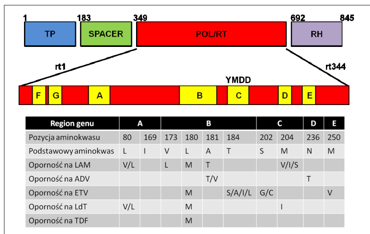
Ryc. 3. Lokalizacja głównych mutacji związanych z opornością HBV na leczenie analogami nukleozydów/nukleotydu (wg [56])
