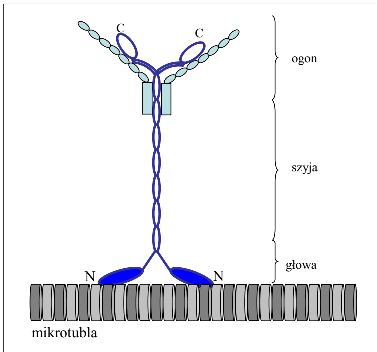
Ryc. 2. Ogólny schemat budowy kinezy z grupy N. Kolorem ciemnoniebieskim oznaczono łańcuchy ciężkie, jasnoniebieskim łańcuchy lekkie
