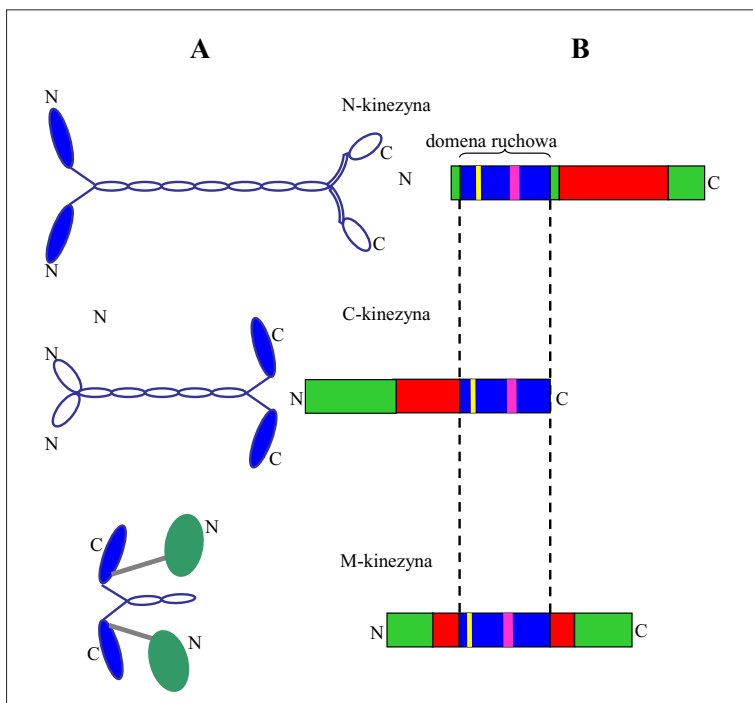
Ryc. 3. Budowa domenowa kinezy; A – modele kinezyn grupy N, C, M, B – struktura białkowa kinezyn grupy N, C, M. Kolor niebieski – domena ruchowa z miejscem wiązania ATP (prostokąt żółty) i miejscem wiązania mikrotubul (prostokąt różowy), kolor czerwony – domena umożliwiająca tworzenie dimerów, zielony – inne domeny o niskim stopniu homologii
